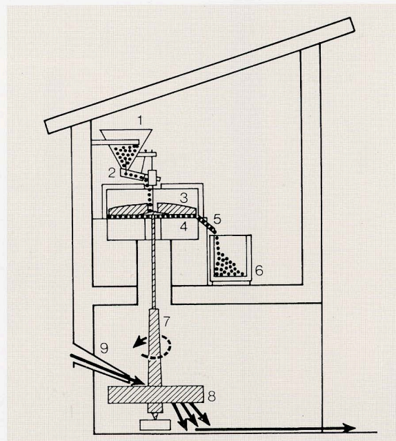
Esquema d'un molí fariner (segons J. Bolòs i J. Nuet, Els molins fariners a Catalunya ).
